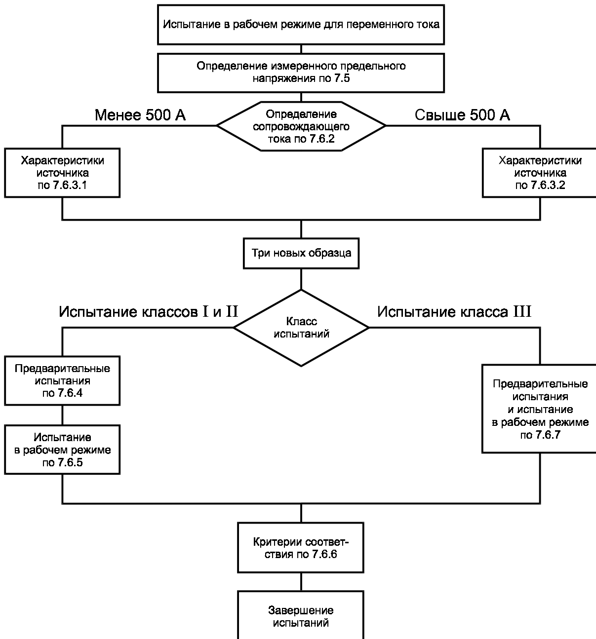
Рисунок 5 — Схема испытания в рабочем режиме
