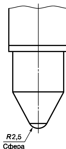
Рисунок 12б — Нагрузочный стержень для испытания давлением шарика
