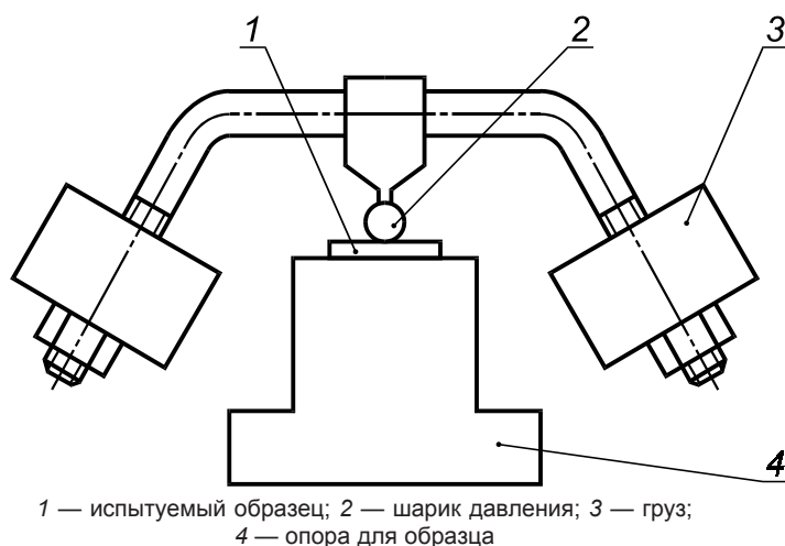
Рисунок 12а — Установка для испытания давлением шарика
