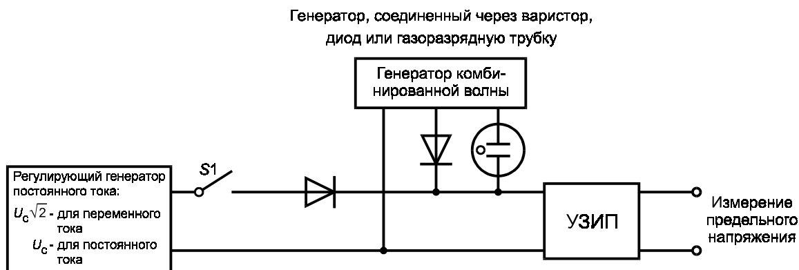
Рисунок 4 — Альтернативное испытание на измеренное предельное напряжение
