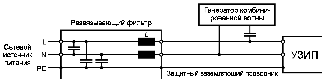
Рисунок 1 — Пример развязывающего фильтра для однофазной сети
